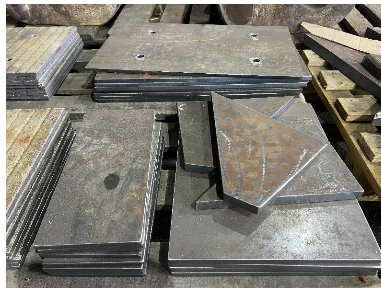
Plazma rezanje, ugljični čelik, debljina 12 mm
